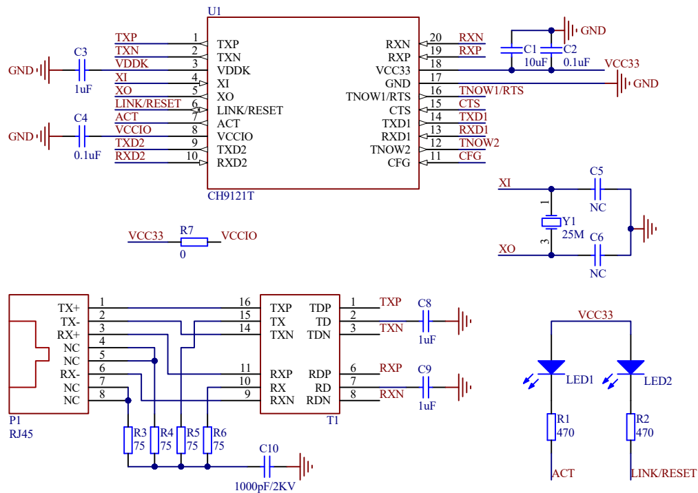
图 9-1 CH9121T 硬件参考电路
